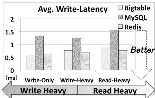
図 5 ストレージエンジンごとの書き込み遅延 Fig. 5 Write latency for each storage engine
