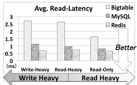
図 6 ストレージエンジンごとの読み出し遅延 Fig. 6 Read latency for each storage engine
