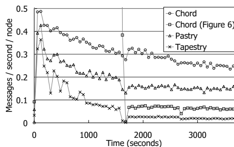
図 10 実機 197 台での 1 秒・1 ノードあたりのメッセージ数 (Recursive ルーティングの場合)
