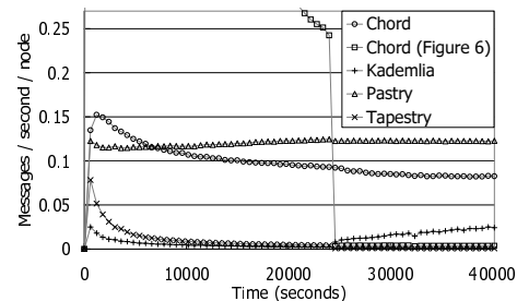
図 7 4000 ノードのエミュレーションシナリオでの 1 秒・1 ノードあたりのメッセージ数 (Iterative ルーティングの場合)
