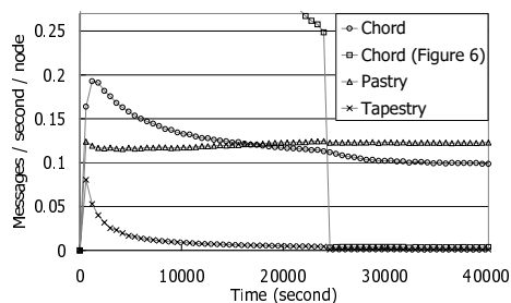
図 8 4000 ノードのエミュレーションシナリオでの 1 秒・1 ノードあたりのメッセージ数 (Recursive ルーティングの場合) Fig. 8 Number of messages per second per node passed between emulated 4000 nodes (recursive routing).
