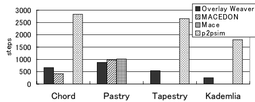
図 6 各アルゴリズム実装のステップ数
