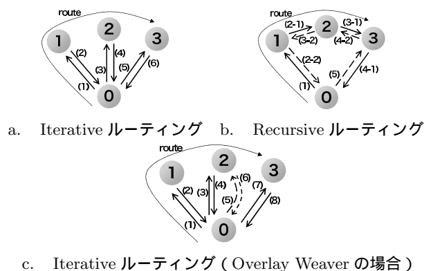
図 3 ルーティングの様式 Fig. 3 Routing styles.
